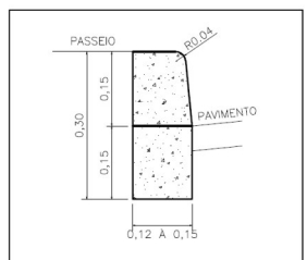
DETALHE DO MEIO-FIO SIMPLES ESC. 1:10
